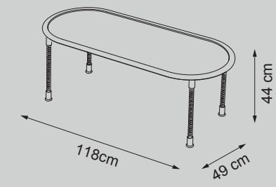
Item D12 table
