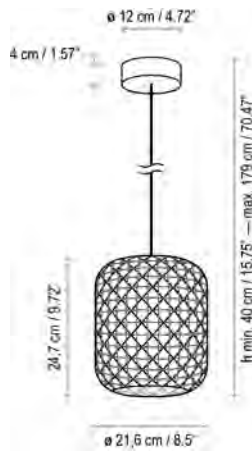
Nans S /21 IP-66
