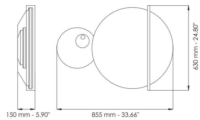
Art. 7500/PL85
